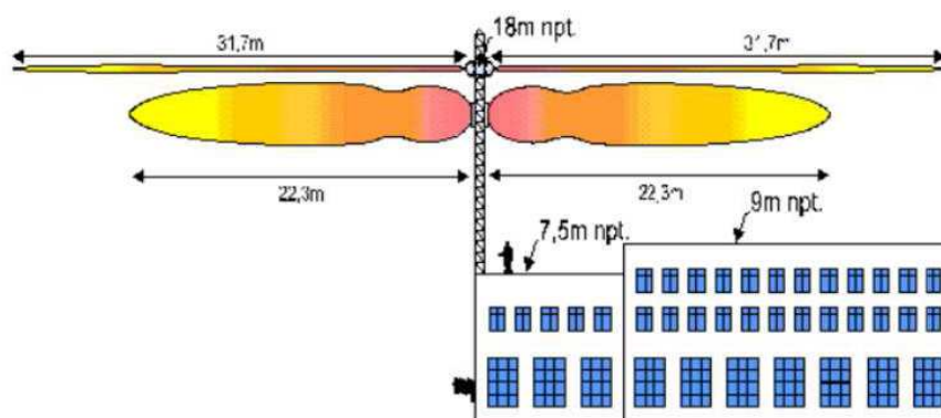
Rys. 22. Rozkład promieniowanie elektromagnetycznego dla anteny stacji bazowej telefonii komórkowej zlokalizowane na budynku
