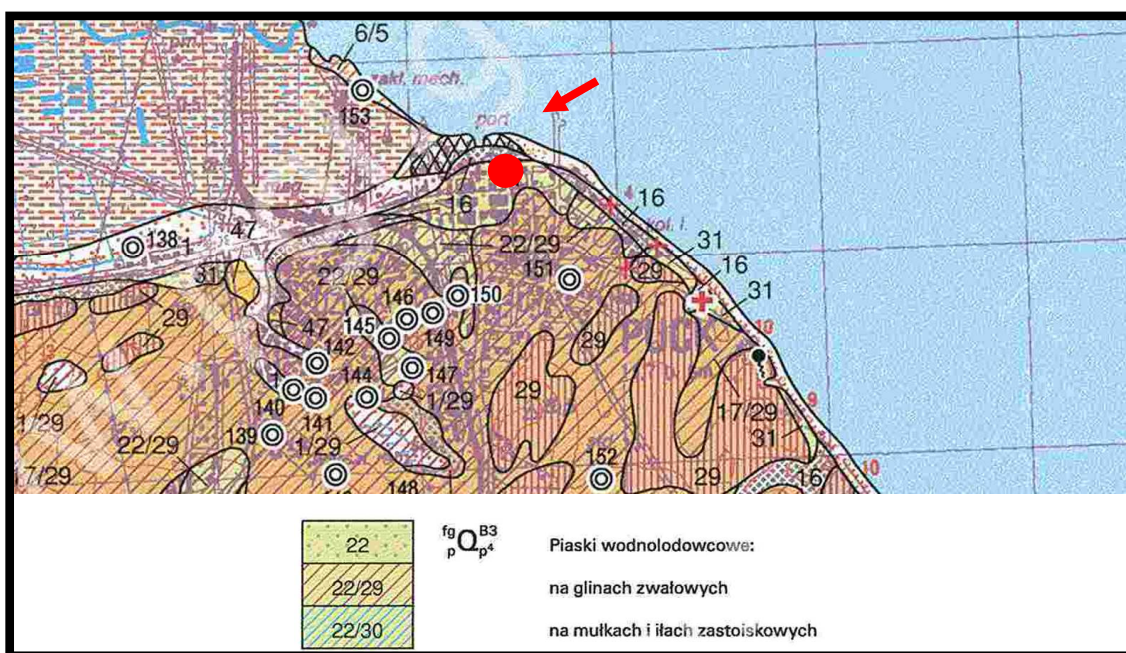
Rys. 19. Ogólna budowa geologiczne terenów w rejonie obszaru objętego projektem planu – lokalizację projektu planu zaznaczono kolorem czerwonym
