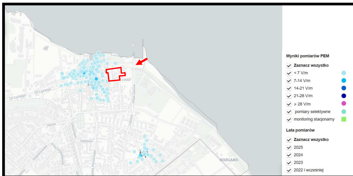
Rys. 23. Wyniki pomiarów pola elektromagnetycznego w rejonie obszaru objętego projektem planu – granice projektu planu zaznaczono kolorem czerwonym
