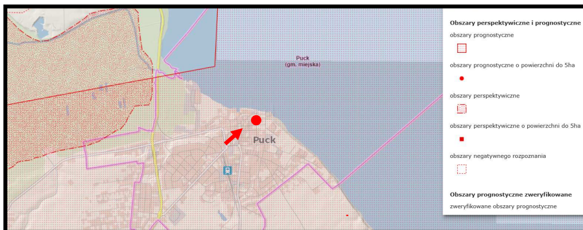
Rys. 28. Położenie obszaru objętego projektem planu w granicach prognostycznych złóż soli kamiennych „Zatoka Pucka” – lokalizację projektu planu zaznaczono kolorem czerwonym
