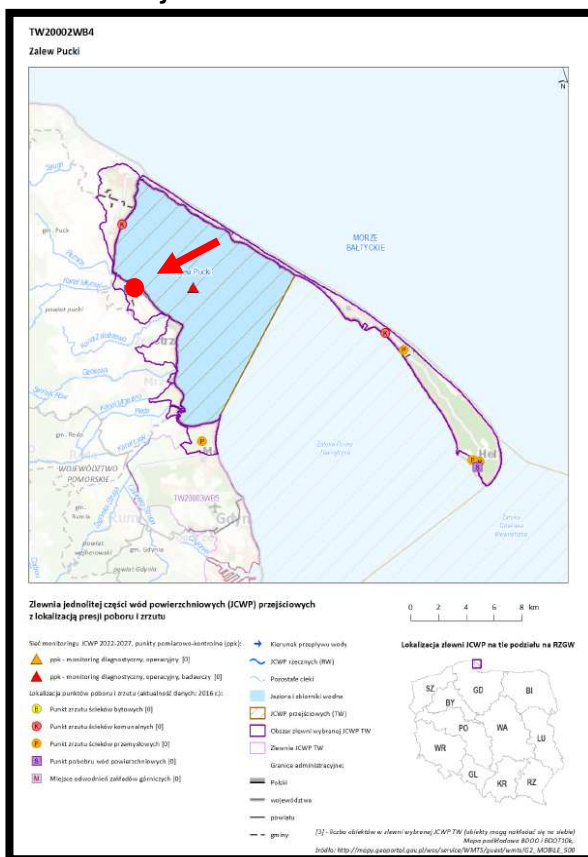
Rys. 16. Położenie obszaru objętego projektem planu w podziale obszaru Polski na jednolite części wód powierzchniowych w granicach JCWP przejściowych JCWP TW20002WB4 Zalew Pucki – lokalizację projektu planu zaznaczono kolorem czerwonym
